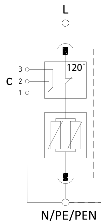
Принципиальная схема
