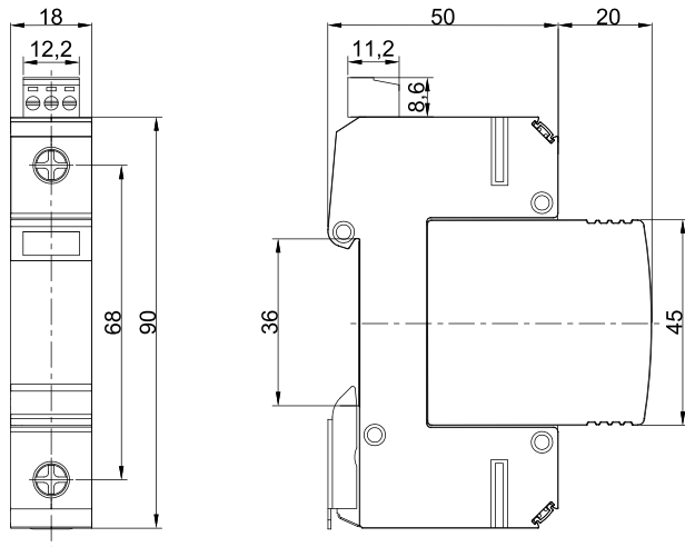
Габаритные размеры
